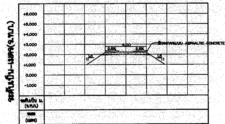
รูปตัดตามขวาง กม.0+075 ขนาดส่วน { ด้านตั้ง 1:100 ด้านราบ 1:100
