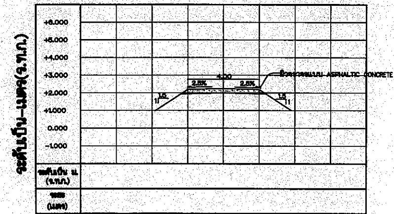
รูปตัดตามขวาง กม.0+285
