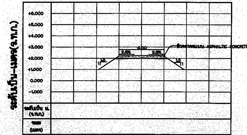
รูปตัดตามขวาง กม.0+150
