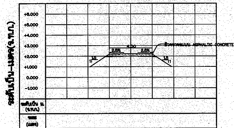
รูปตัดตามขวาง กม.0+275
