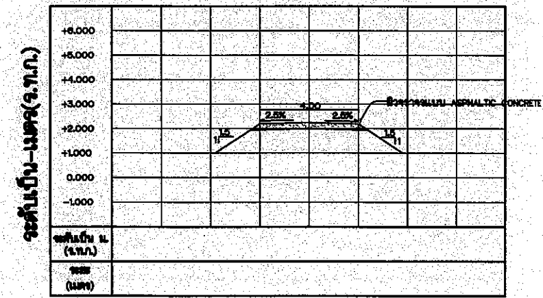
รูปตัดตามขวาง กม.0+100 ขนาดส่วน { ด้านตั้ง 1:100 ด้านราบ 1:100
