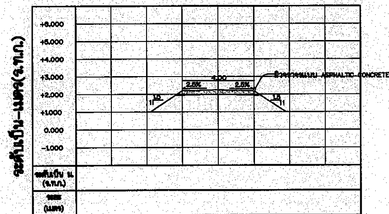
รูปตัดตามขวาง กม.0+175
