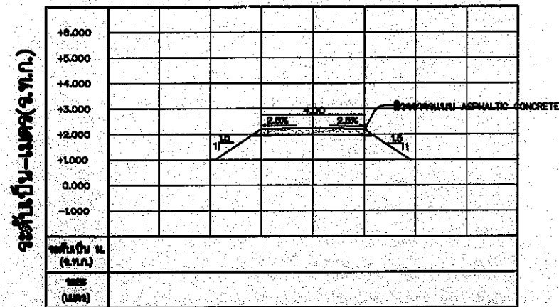
รูปตัดตามขวาง กม.0+125
