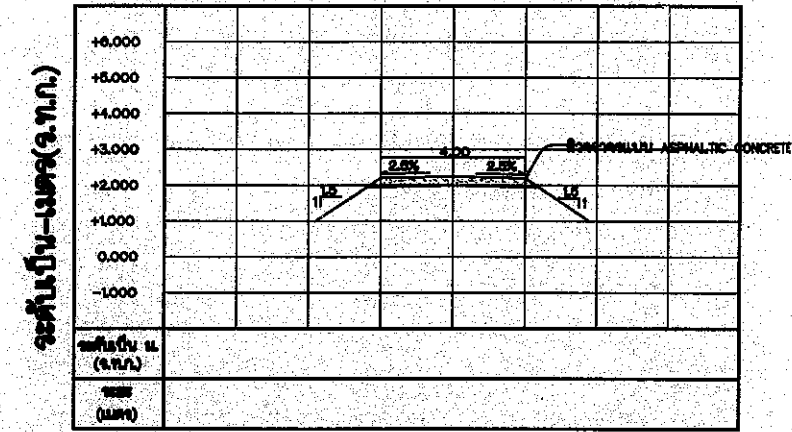
รูปตัดตามขวาง กม.0+050 ขนาดส่วน { ด้านตั้ง 1:100 ด้านราบ 1:100
