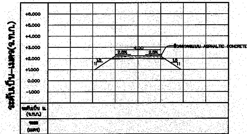
รูปตัดตามขวาง กม.0+225
