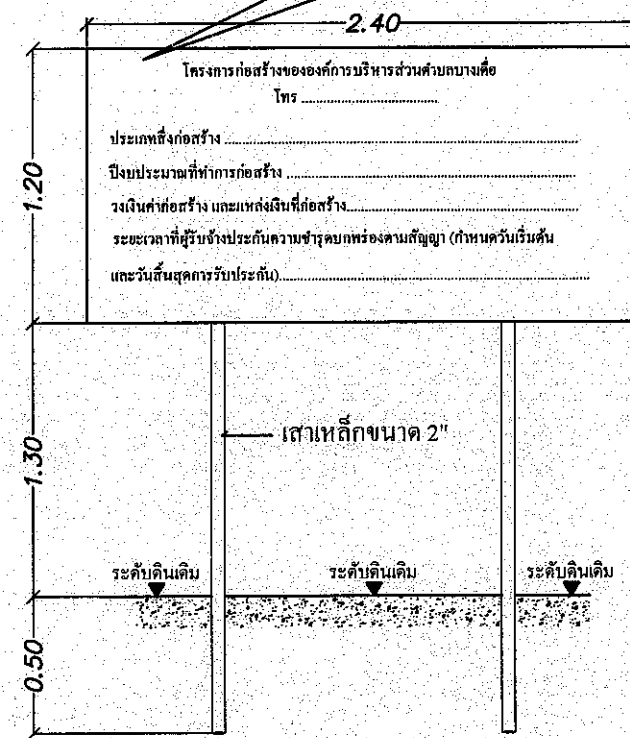
แบบป้ายโครงการถาวร
